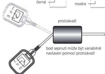
Champ – rozměry, schéma zapojení
