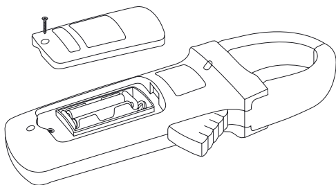
Bild 7: Batteriewechsel Fig. 7: Battery replacement Fig. 7: Remplacement de la pile Fig. 7: Cambio de batería obr. 7: Výměna baterií σχήμα 7: Αντικατάσταση μπαταρίας ill. 7: Sostituzione batterie Fig. 7: Vervanging van de batterijen Rys. 7: Wymiana baterii Imaginea 7: Schimbarea bateriilor рис. 7: Замена батареи Fig. 7: Batteribyte Resim 7: Batarya Değişimi
