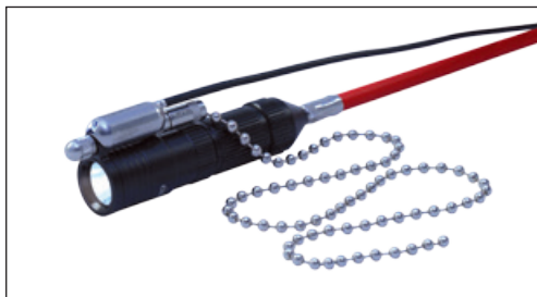
RUNPOCAM s kuličkovým řetězkem – akumulátorová LED svítilna – produkty RUNPOTEC se závitem RTG Ø 6 mm.
