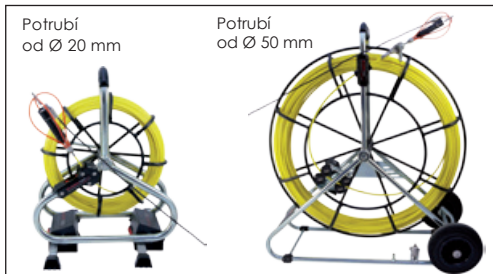
Pro inspekci potrubí. Pera ze skelných vláken Ø 3 mm, Ø 4,5 mm, Ø 6 mm nebo Ø 7,5 mm, Ø 9 mm, Ø 11 mm a Ø 15 mm s kombinací RUNPOCAM
